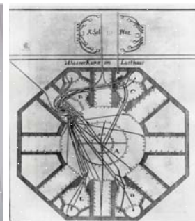
J. van den Nypoort, Půdorys Rotundy s vodním strojem, 1691
